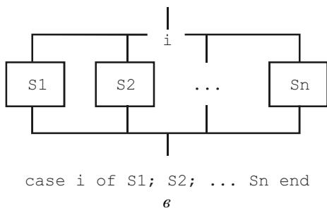
Рис. 5.5. Структура "альтернатива".
