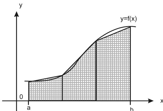
Рис. 6.20. Численное интегрирование методом трапеций
