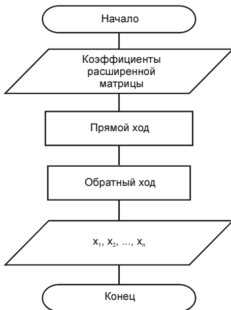
Рис. 6.13. Блок-схема алгоритма метода Гаусса
